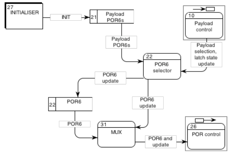
Simulator DFD : POR control
