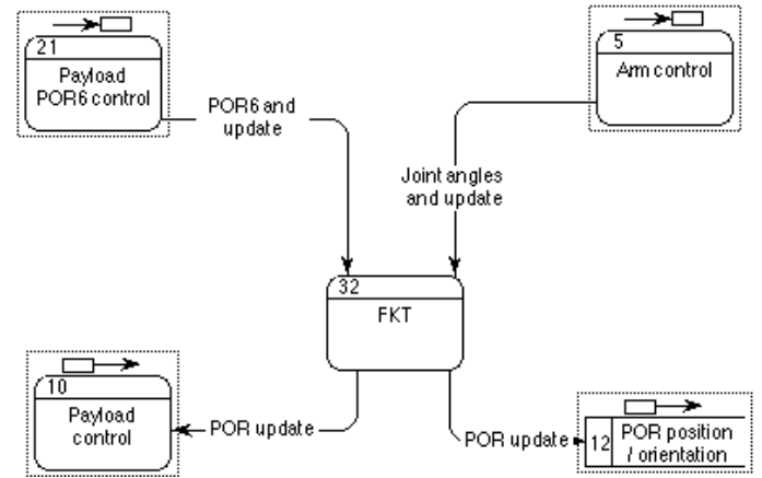
Simulator DFD : POR control
